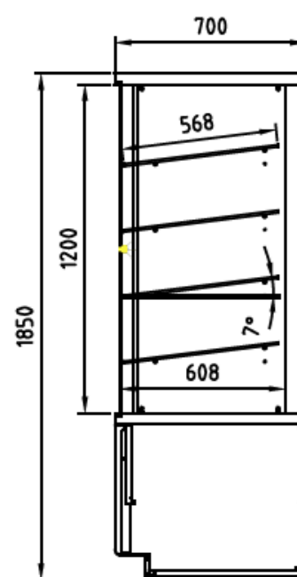
SECCIÓN CMCT-70-RC
