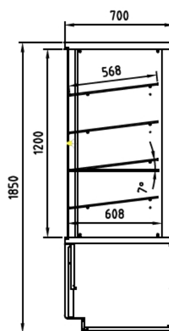
SECCIÓN CMCT-70-RC
